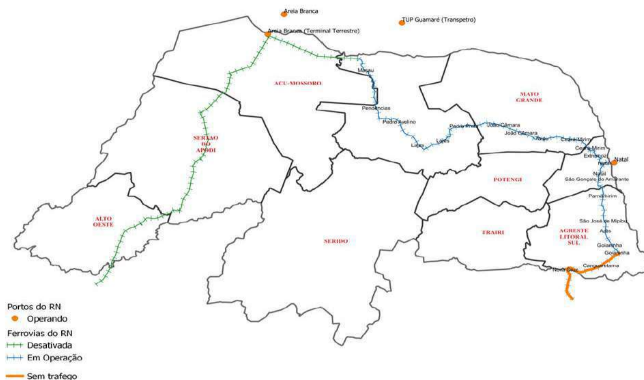
Mapa 35 - Malha ferroviária do Rio Grande do Norte
