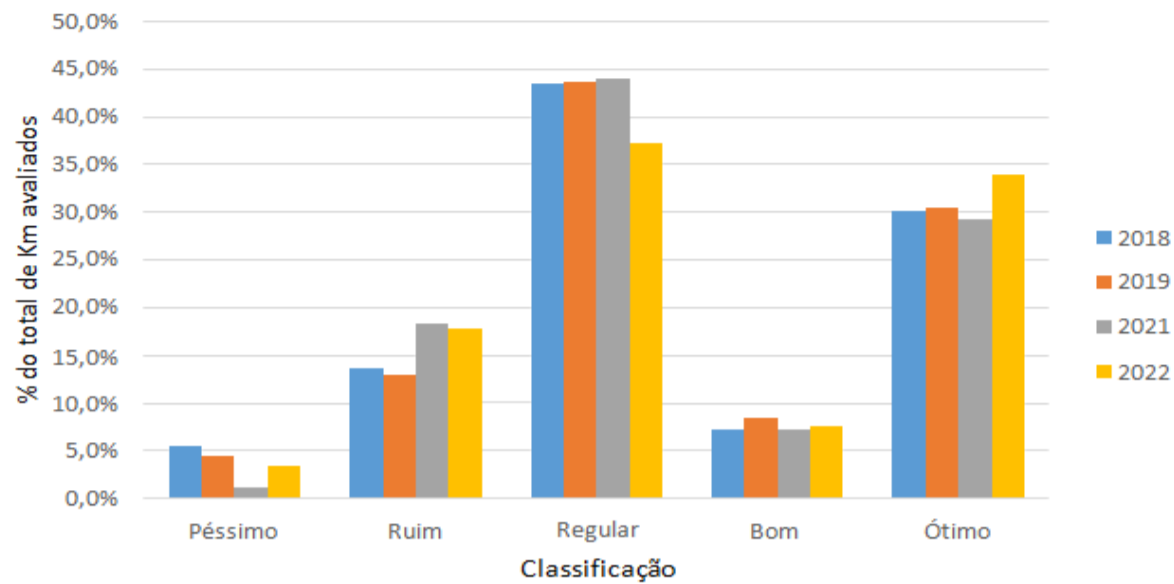
Gráfico 72 - Qualidade do Pavimento das Rodovias do RN (2018-2022)
