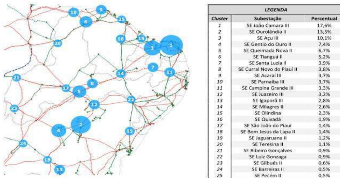
Mapa 24 – Brasil – Representação da expansão indicativa de subestações
