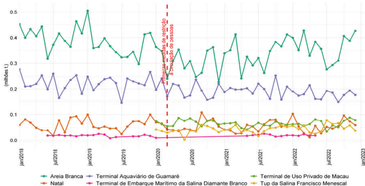
Gráfico 66 – Evolução mensal da movimentação portuária (milhões de toneladas). Rio Grande do Norte, 2018 e 2022
